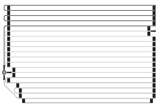
Trippelflöde
